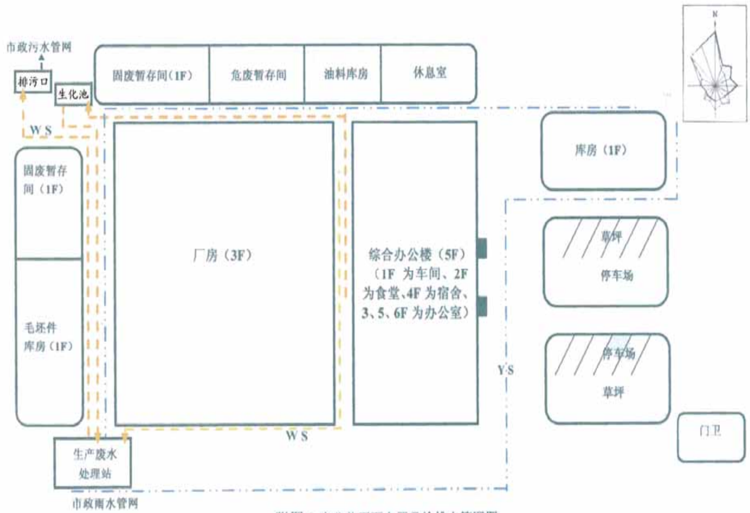
附图 2 企业总平面布置及给排水管网图
