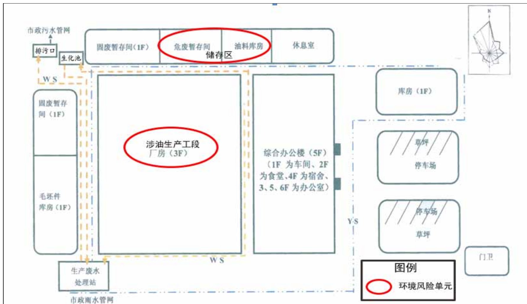
附图3 企业环境风险单元图
